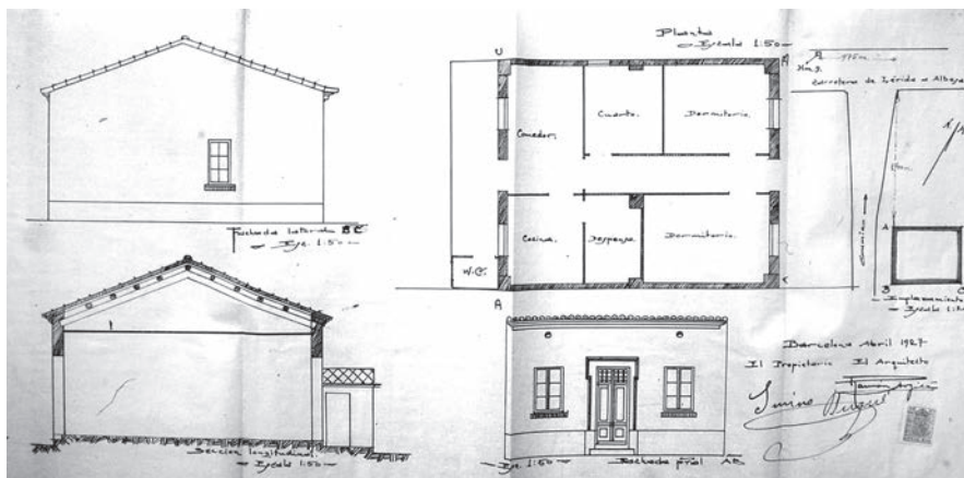
Plànol d'un projecte de casa presentat a l'Ajuntament de Lleida, el 1927. Font: Arxiu Municipal de Lleida. Secció Administrativa.
