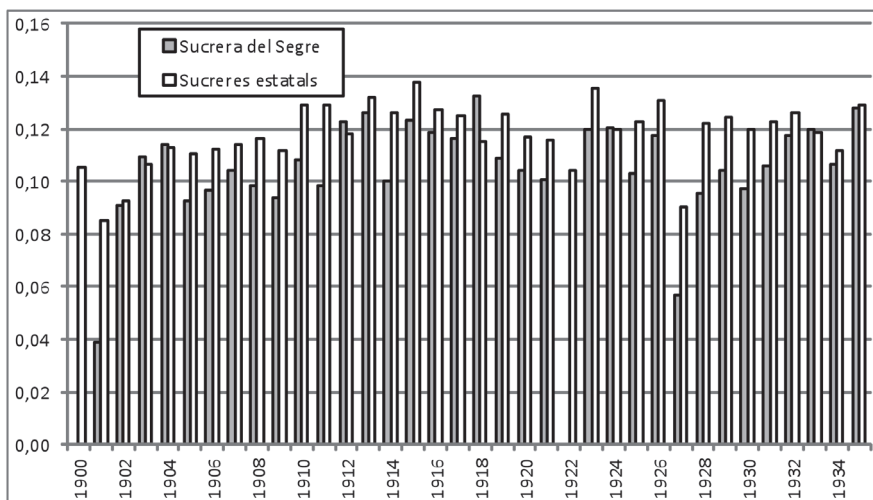
GRÀFIC 4 RENDIMENTS DE LA SUCRERA DEL SEGRE I DEL CONJUNT DE LES SUCRERES ESTATALS (KG SUCRE / KG REMOLATXA), 1899/1900-1934/1935
