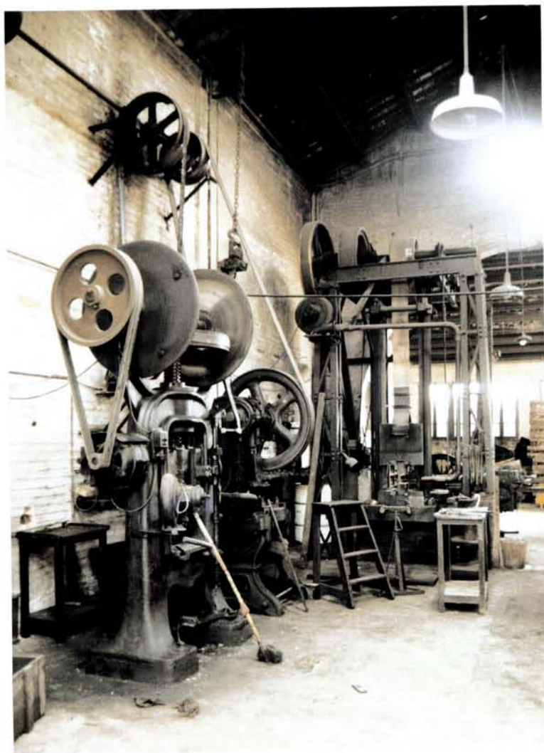
Nau número 10. Detall d'unes estampes que es feien i s'utilitzaven en aquesta nau. Any 1995. (Fotografia: Oriol Saula. AFMCUT)
