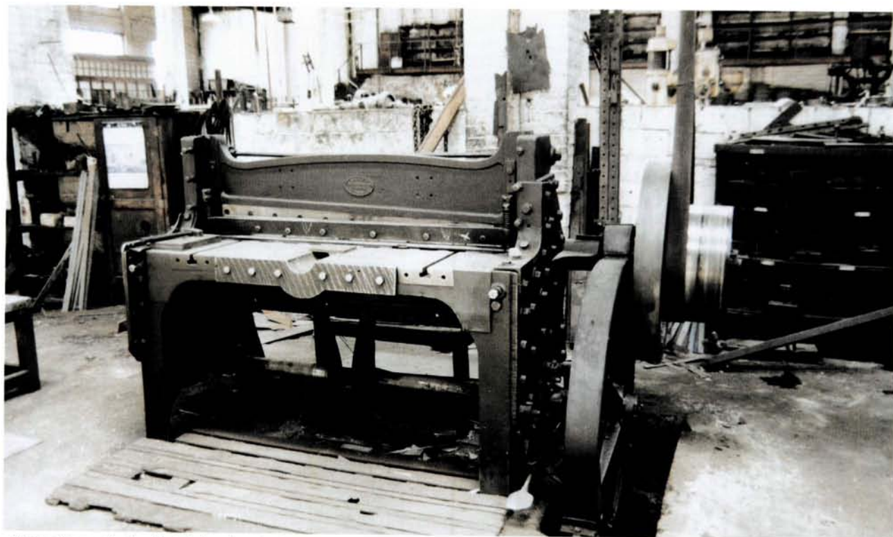
Nau número 6. Cisalla fabricada a la ciutat anglesa de Manchester. Fixeu-vos que totes les peces de la màquina estan fixades amb cargols i femelles. Any 1995. (Fotografia: Oriol Saula. AFMCUT)
