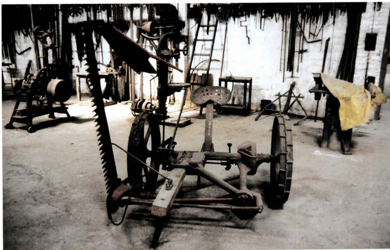
Màquina dalladora Mc Cormick, importada dels Estats Units, a la fàbrica J. Trepà. Any 1995. (Fotografia: Oriol Saula; Arxiu Fotogràfic del Museu Comarcal de l'Urgell, Tàrraga. AFMCUT)
