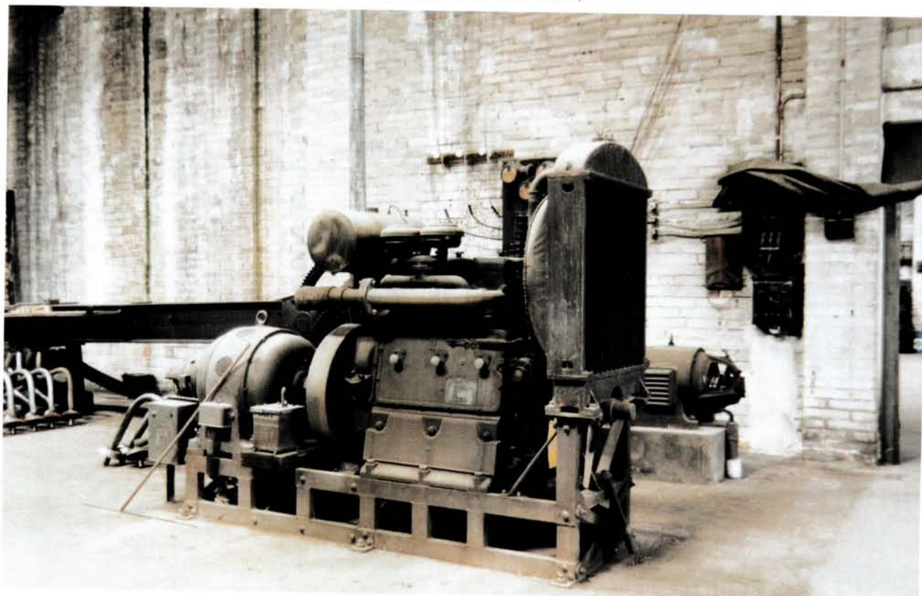
Nau número 10. Motor de tres cilindres amb dinamo per produir llum en cas de restricció elèctrica. Any 1995. (Fotografia: Oriol Saula, AFMCUT)
