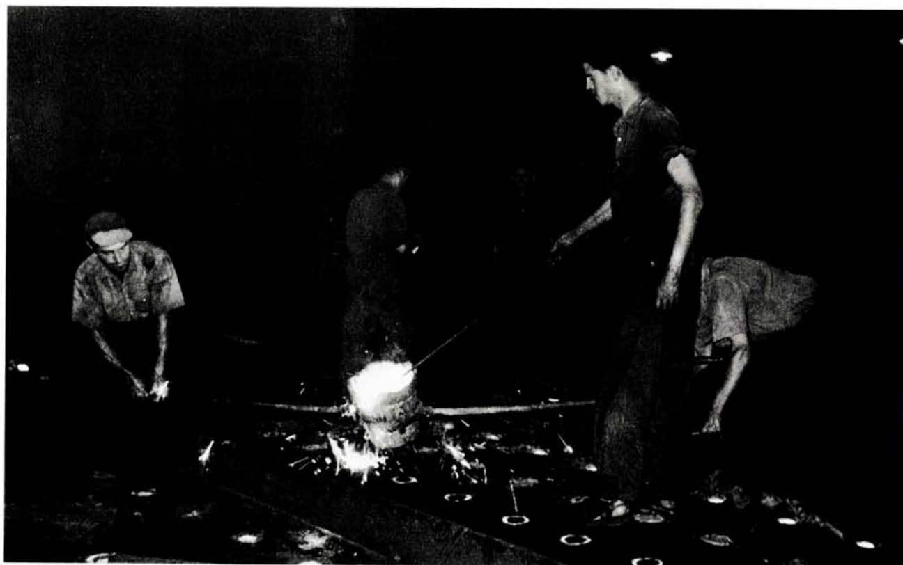
Secció de Foneria. S'omplen els motlles de les peces amb el ferro fos. Dia 21 de setembre de 1957. (Fotografia: Calafell. Arxiu Fotogràfic Comarcal de l'Urgell. AHCT).
