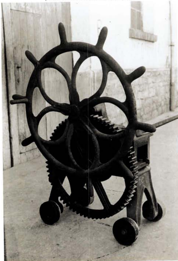
En aquestes tres imatges veiem una màquina de foradar, una màquina de corbar i una màquina de recalcar. Aquestes tres màquines es van produir a la fàbrica J. Trepà per a ús propi, però posteriorment es van comercialitzar per als ferrers i els representants que l'empresa tenia per tot el país. (Arxiu de les Indústries J. Trepà)
