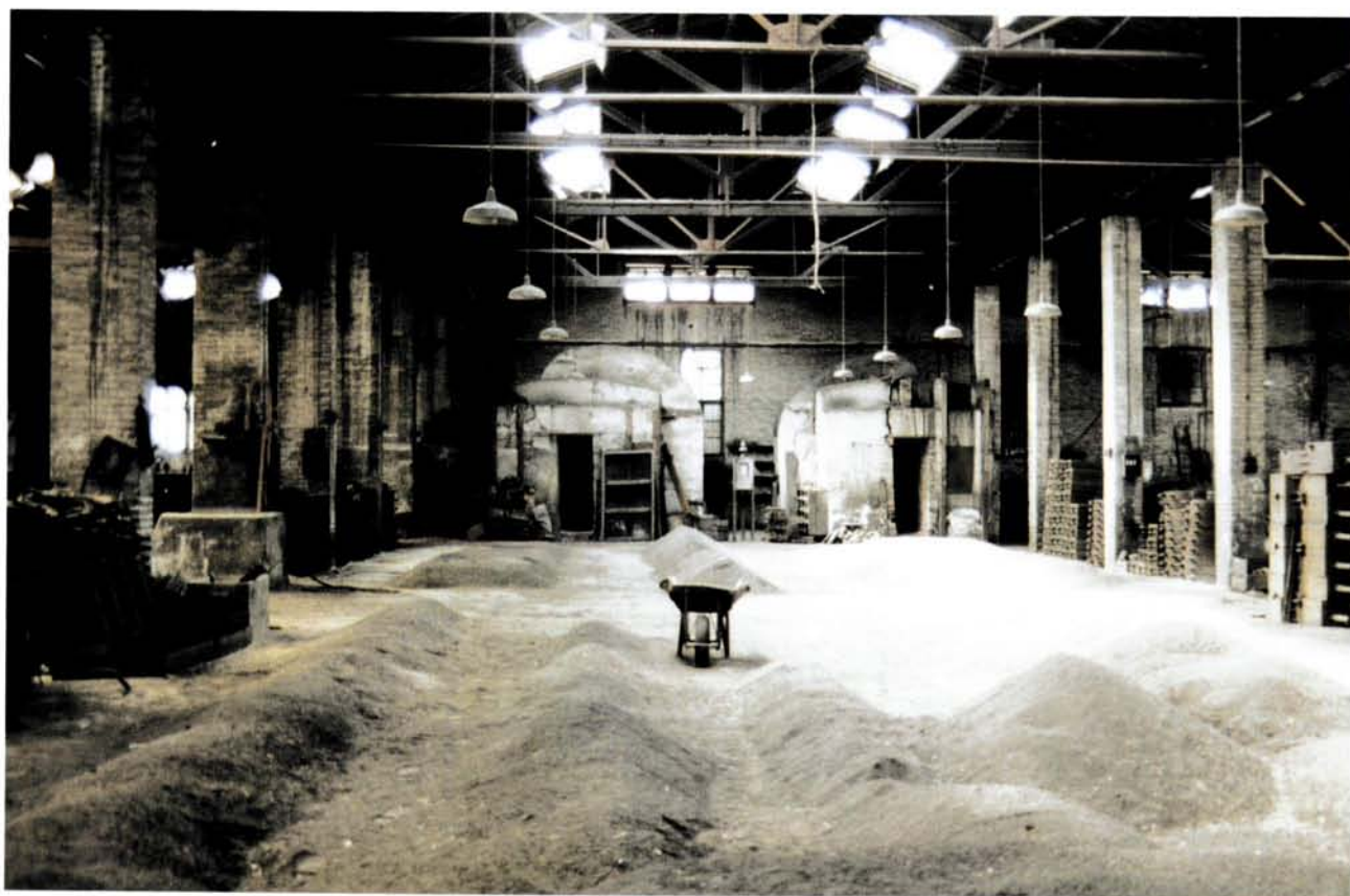
Nau número 2. Al fons de la imatge, el forn de ferro colat manejable. Any 1995. (Fotografia: Oriol Saula. AFMCUT)
