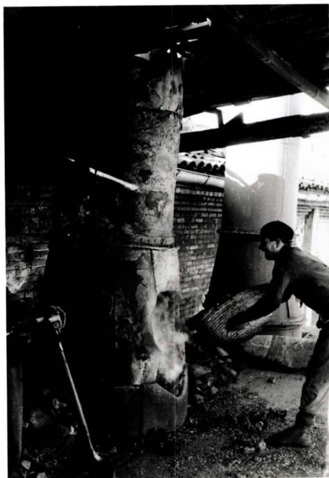
Secció de foneria, càrrega del cubilot. Anys 50. (Arxiu de les indústries J. Trepal)
