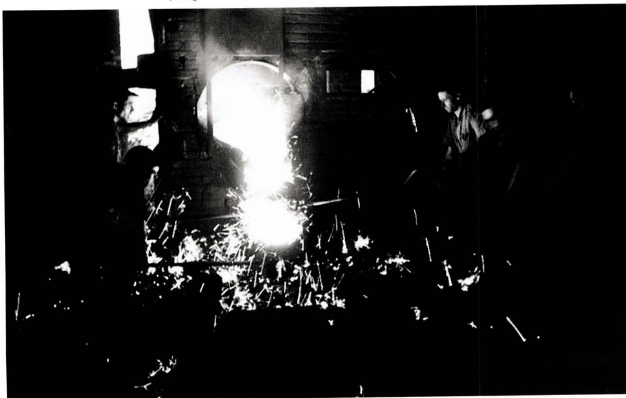
Secció de Foneria. Descàrrega del cubilot una vegada s'ha fos el ferro. Dia 21 de setembre de 1957. (Fotografia: Calafell. Arxiu fotogràfic Comarcal de l'Urgell AHCT)
