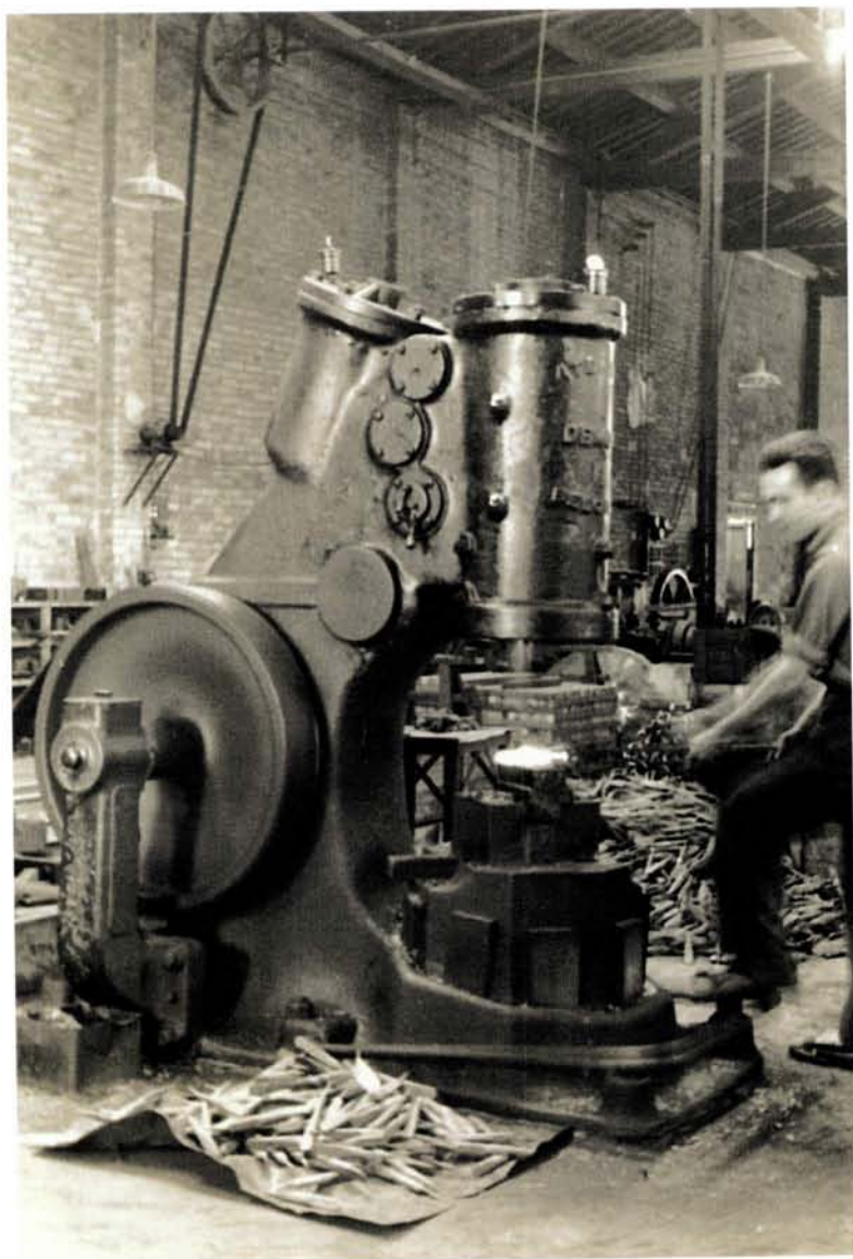
Nau número 10. Treballador fent funcionar el martell piló. Anys 1961-62. (Arxiu de les Indústries J. Trepat)
