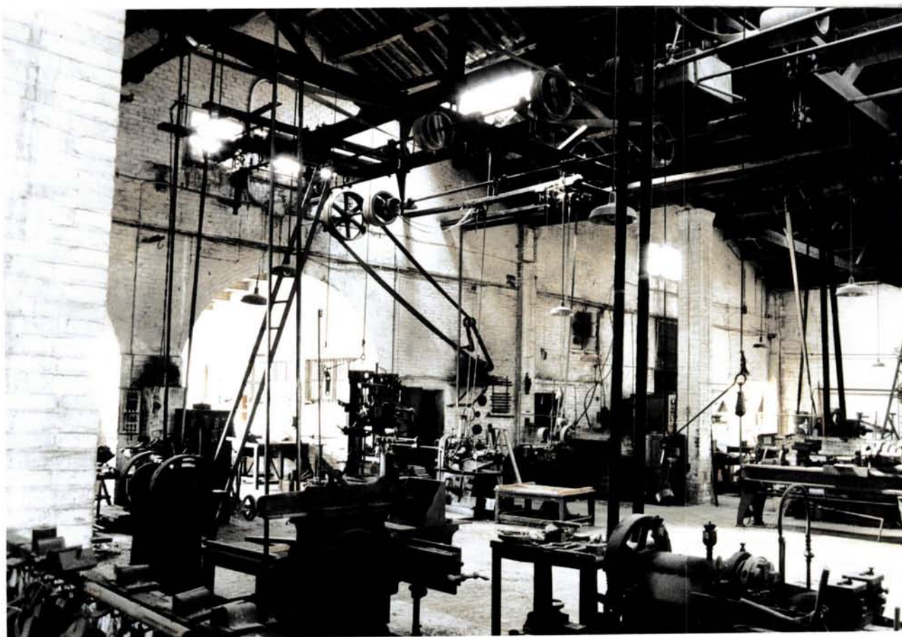
Naus números 5 i 6. Observeu l'espectacular embarrat. Any 1995. (Fotografia: Oriol Saula. AFMCUT)
