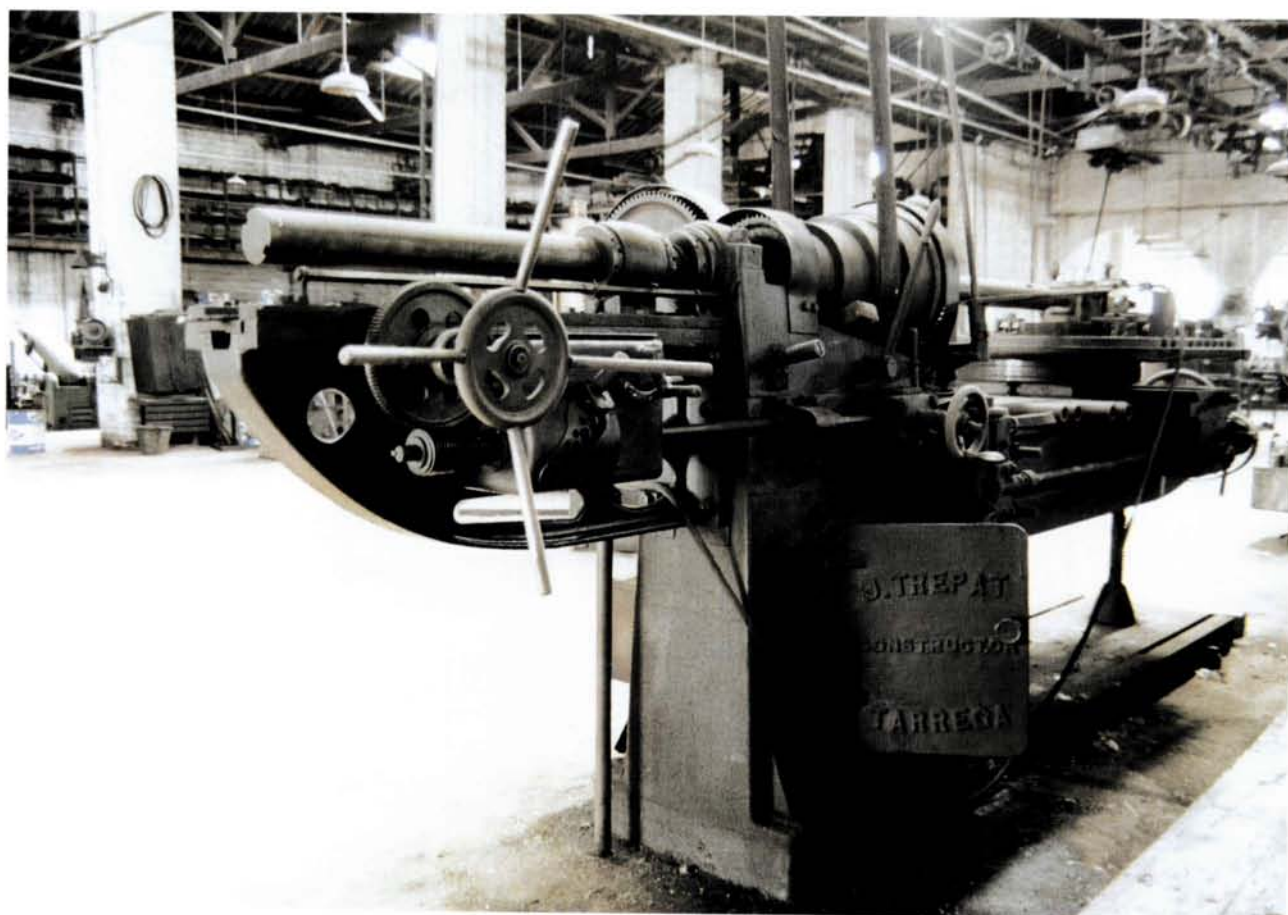
Nau número 5. Màquina mandrinadora que servia per fer els forats horitzontals a les bancades de les dalladores. Any 1995. (Fotografia: Oriol Saula. AFMCUT)
