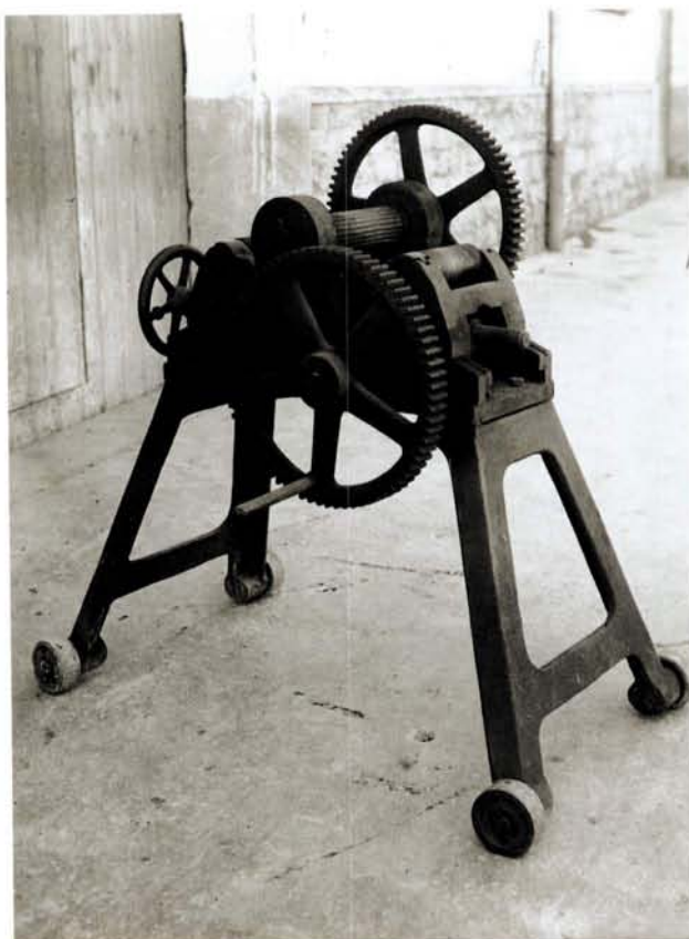
En aquestes tres imatges veiem una màquina de foradar, una màquina de corbar i una màquina de recalcar. Aquestes tres màquines es van produir a la fàbrica J. Trepà per a ús propi, però posteriorment es van comercialitzar per als ferrers i els representants que l'empresa tenia per tot el país. (Arxiu de les Indústries J. Trepà)
