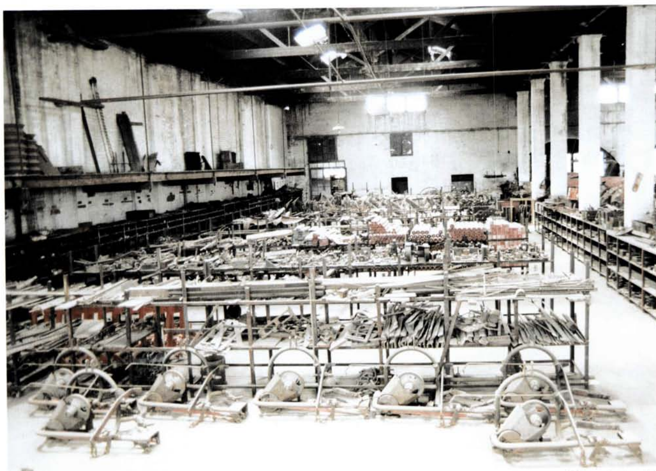
Nau número 11. Secció de Lligadores. A la imatge veiem els estris i les peces de les màquines lligadores. Al fons, la Secció de Lones. Any 1995. (Fotografia: Oriol Saula. AFMCUT)
