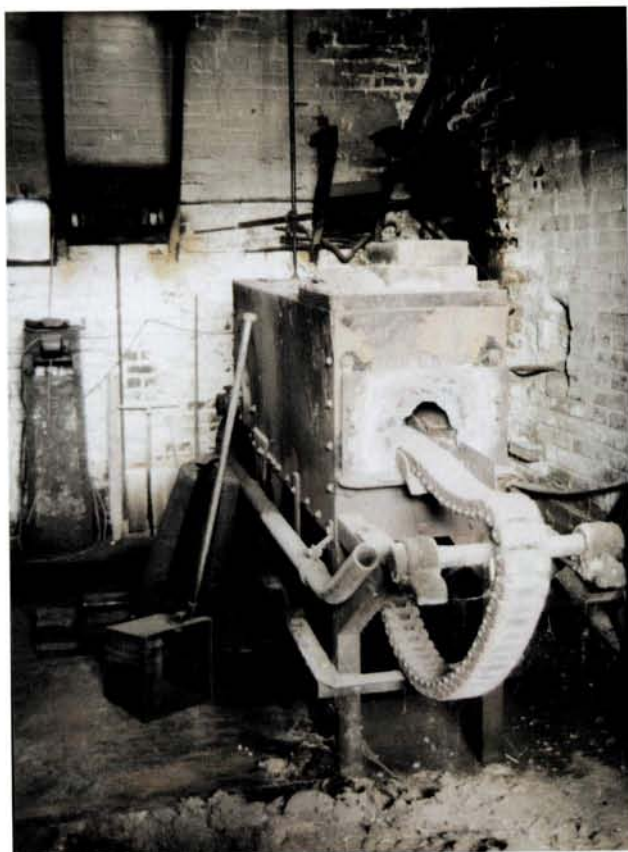
Nau número 6. Al fons trobem el forn de trempar els tallants de les segadores. Funciona a base d'un cremador de gasoil. L'accionament de la cadena alimentadora és elèctric. Any 1995. (Fotografia: Oriol Saula. AFMCUT)
