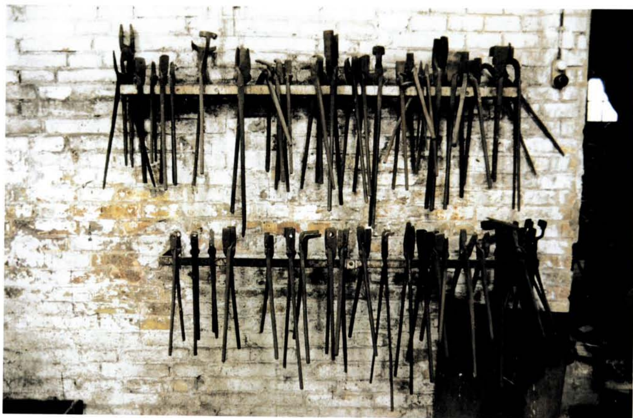
Nau número 9. Detall de les estenalles utilitzades pels forjadors. Any 1995. (Fotografia: Oriol Saula. AFMCUT)
