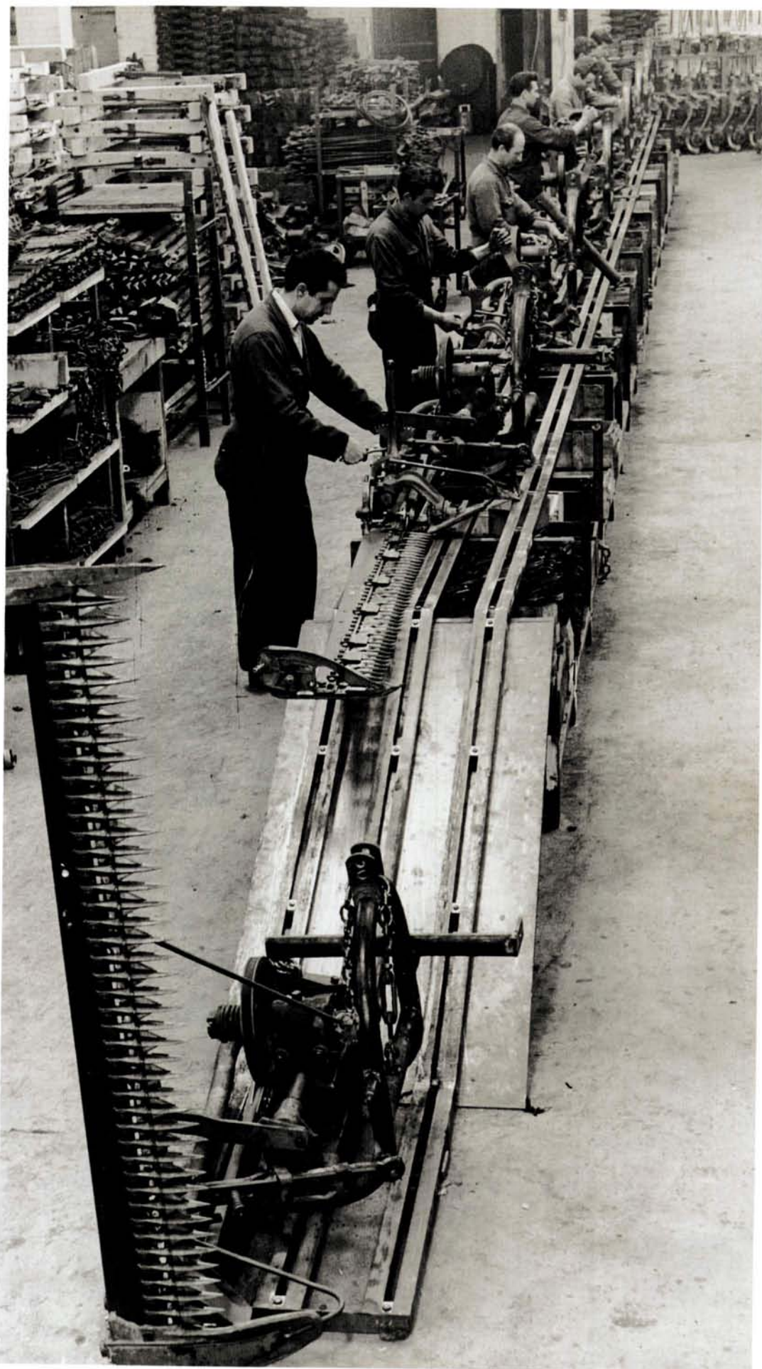
Nau número 9. Els treballadors de la cadena en ple muntatge de les màquines segadores d'alfals per a tractor. Anys 1961-62. (Fotografia: Calafell. Arxiu de les Indústries J. Trepà)
