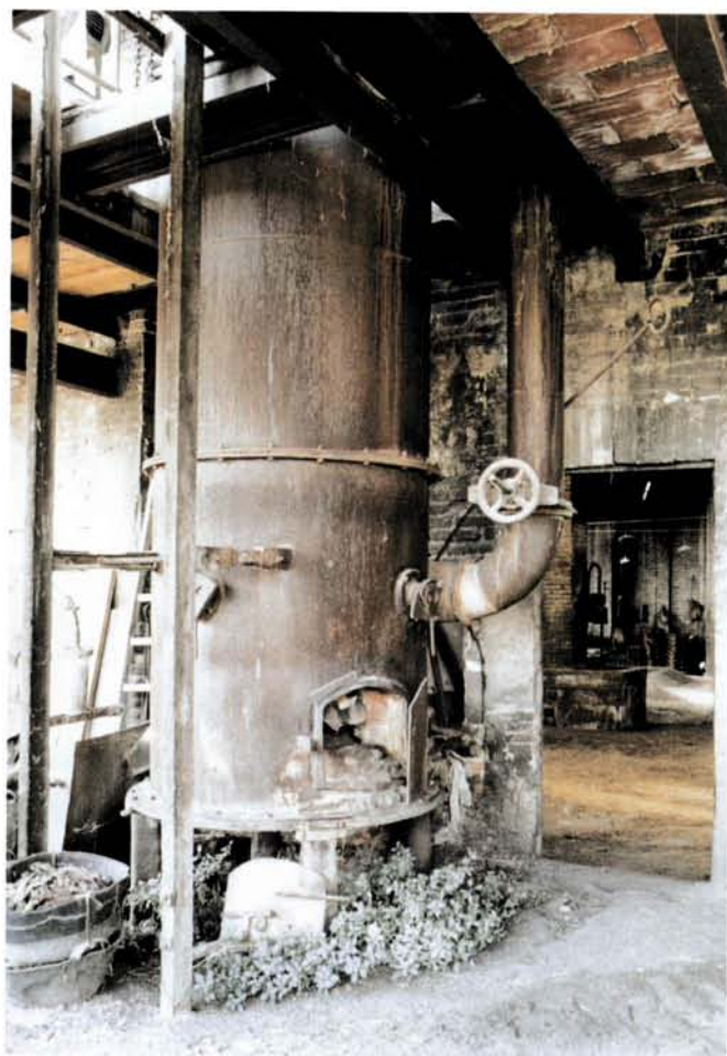
Nau número 1. Foneria. Any 1995. (Fotografia: Oriol Saula. AFMCUT)
